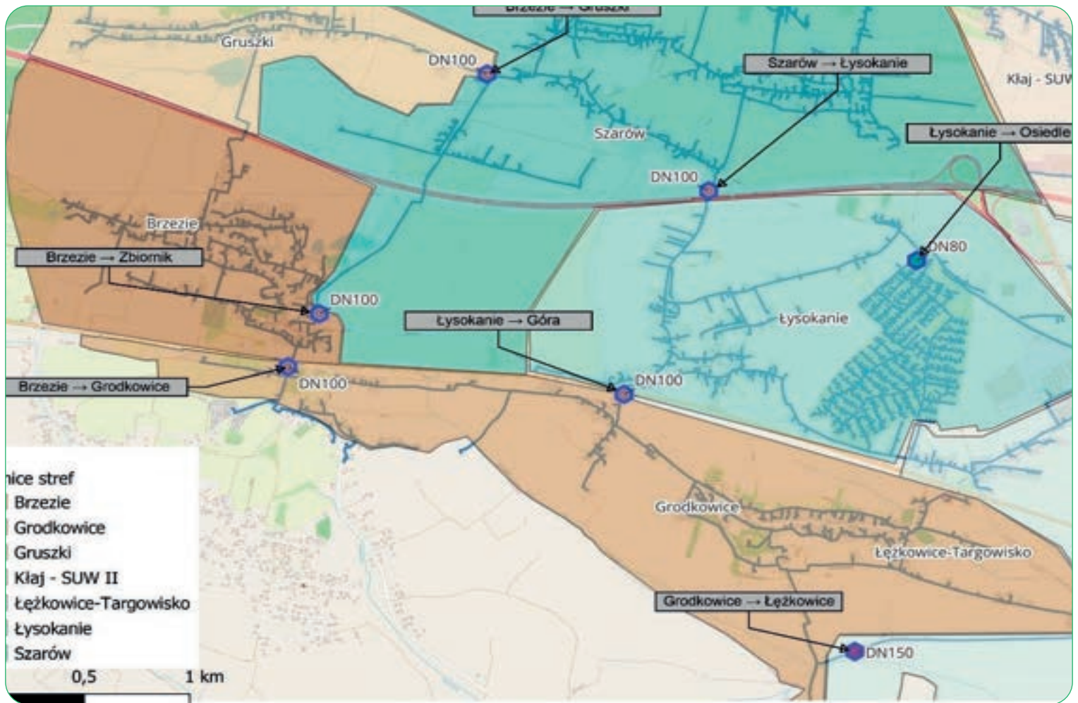
Powstające strefy District Metered Area sieci wodociągowej Gminy Kłaj
